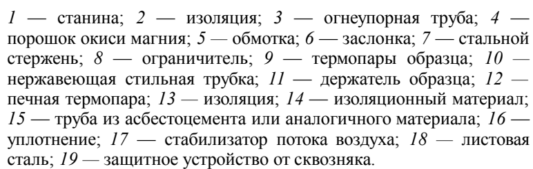
Рисунок А1 — Общий вид установки
